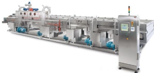
légende de l'image 25 Tunnel de traitement thermique à pluie
